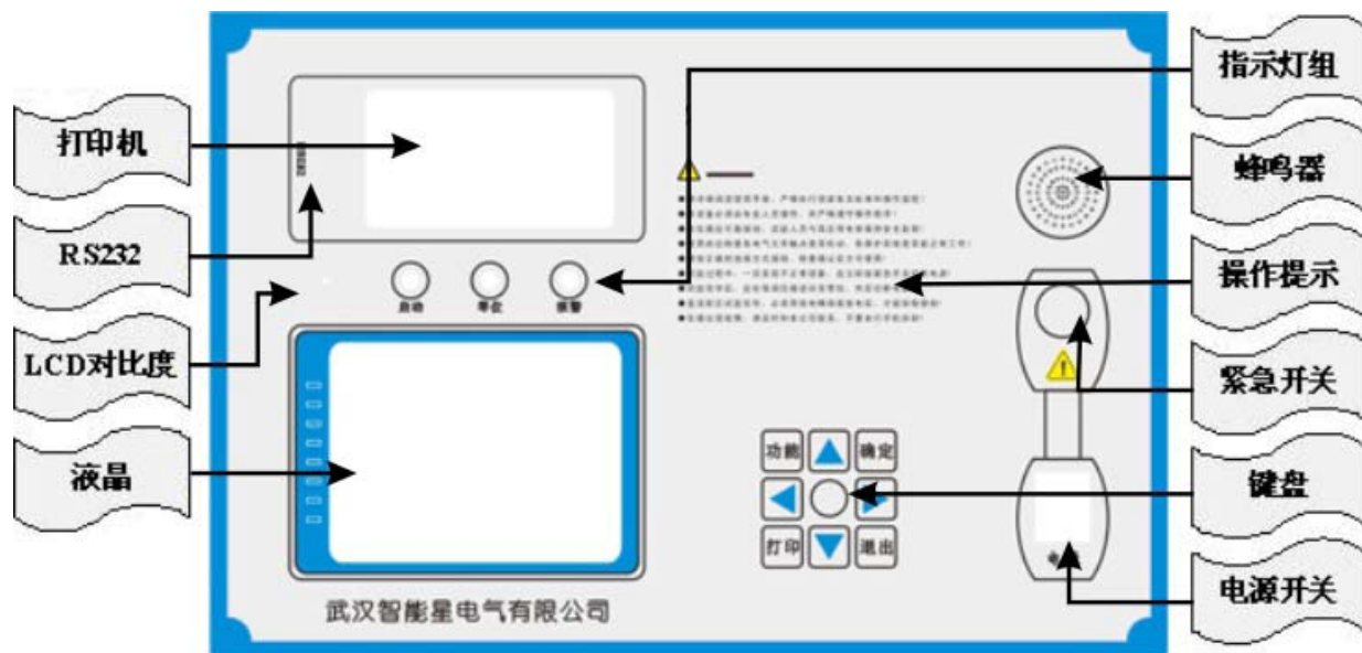
图 2 面板结构图
