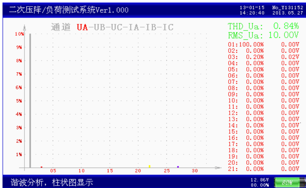
图十八 谐波分析
