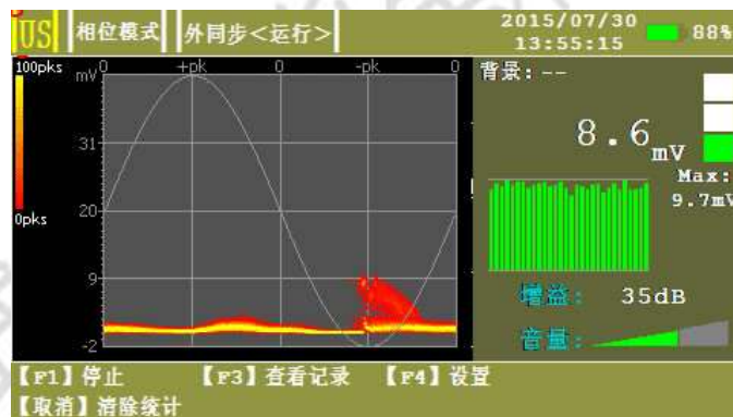
图 0-13 US 相位模式测量画面
