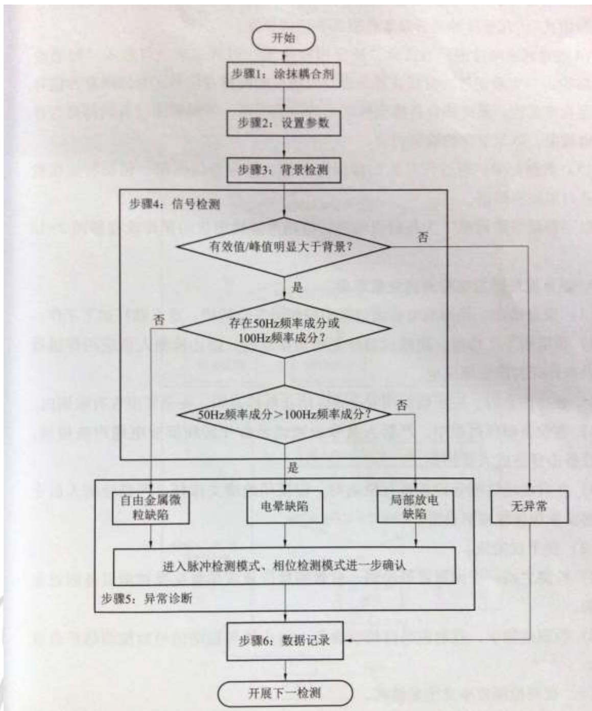
图 0-1 US 检测流程
