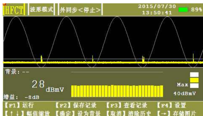
图 0-8 HFCT 波形停止模式
