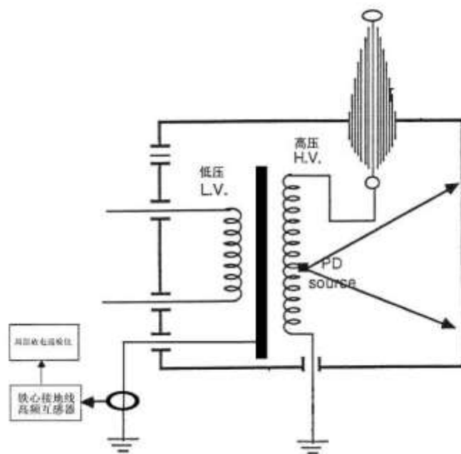
图 0-2 HFCT 变压器检测原理
