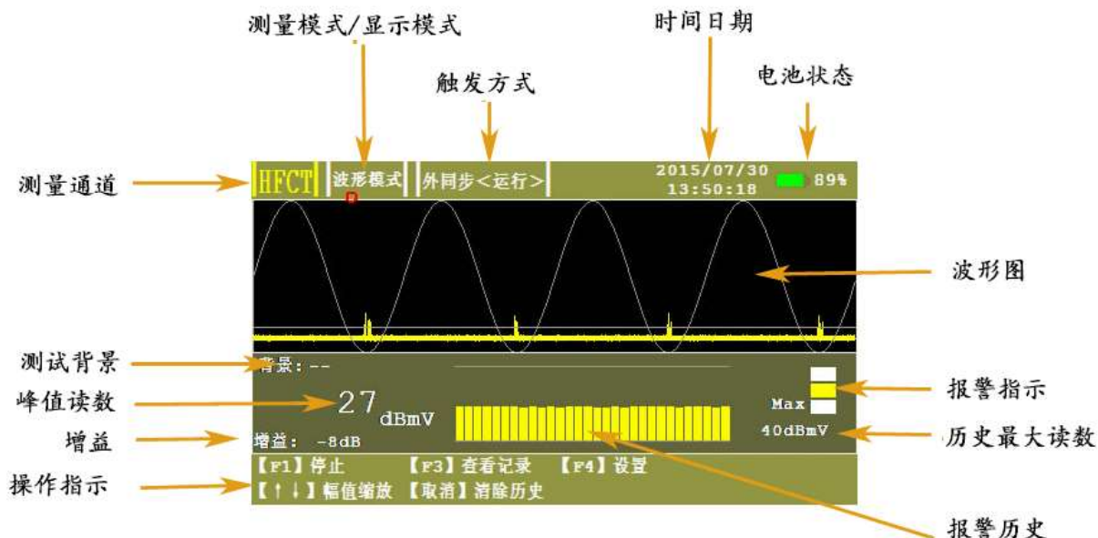
图 0-7 HFCT 波形运行模式
