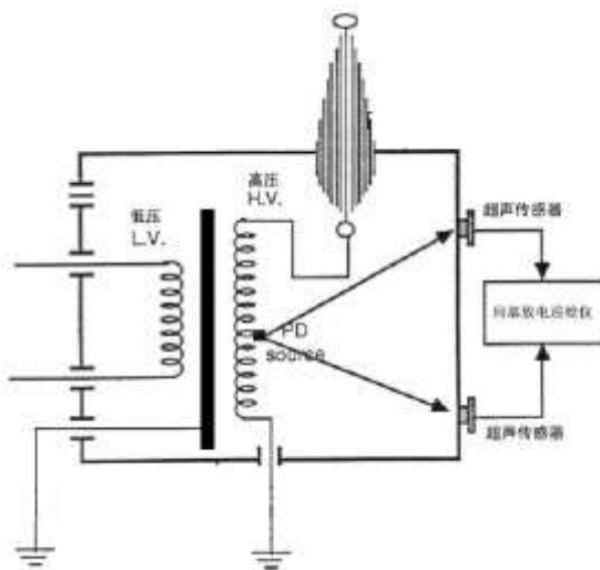
图 0-2 US 变压器检测原理
