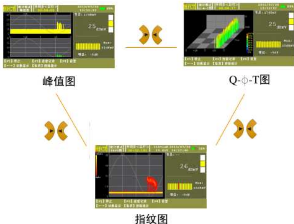
图 0-9 显示模式切换
