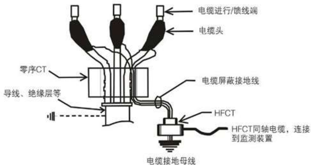
图 0-1 HFCT 电缆检测原理
