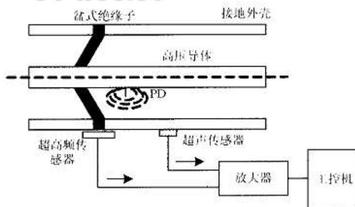
图 6-3 UZ 和超声波联合检测
