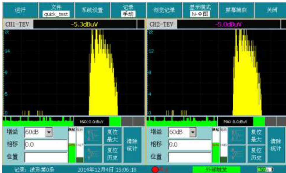
图 4-12 N-Φ图模式
