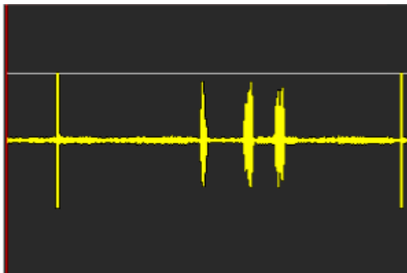
8-6 发生严重放电（电信号）
