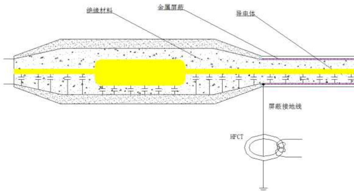
8-1 ZCT 电缆检测原理
