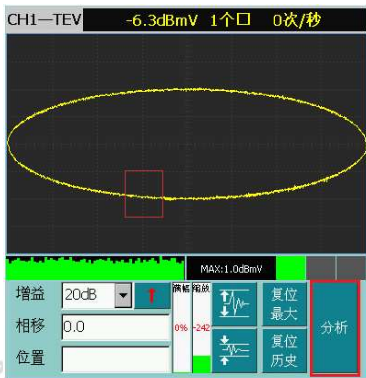
图 4-16 开相位窗并进行单脉冲分析
