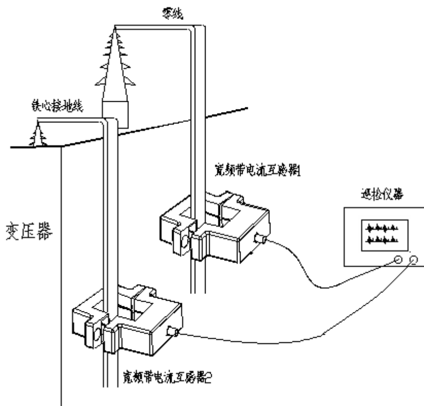
图 7-3 ZCT 检测位置
