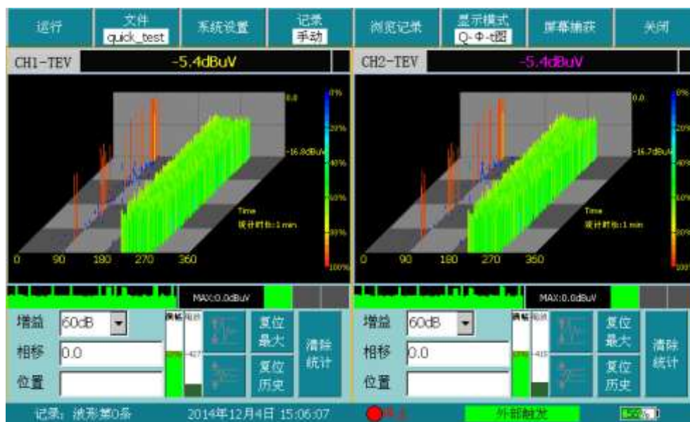
图 4-14 Q-Φ-T 图模式
