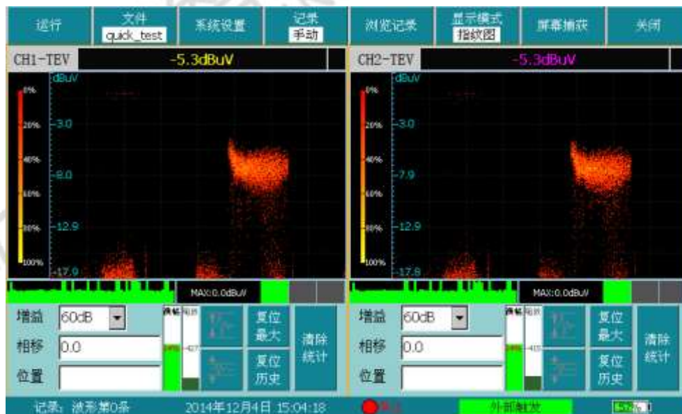
图 4-11 指纹图模式
