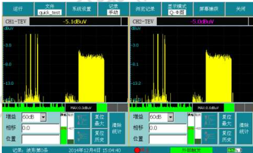
图 4-13 Q-Φ图模式
