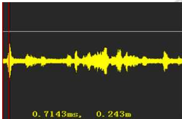
8-7 发生严重放电（声信号）
