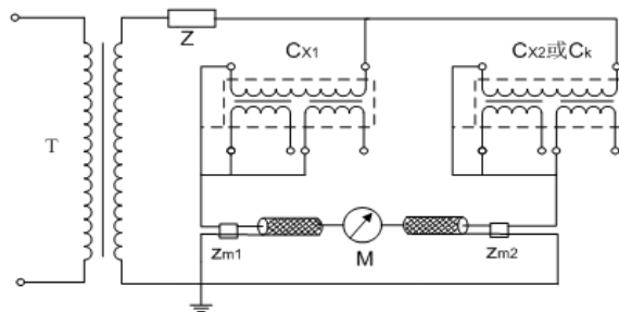
图 5.5 平衡回路
