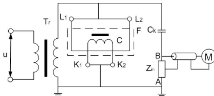
图 5.11 接有耦合电容器 C_k 的试验接线
