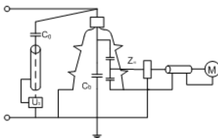
图5.14. C 套管抽头测量和校准接线
