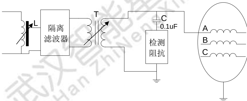
图5.13 发电机的局放测试接线
