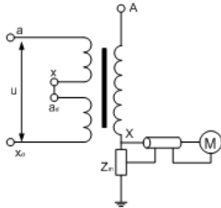
图 5.6 无耦合电容器 G 试验接线
