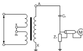
图 5.8 接有耦合电容器 C_k 的试验接线
