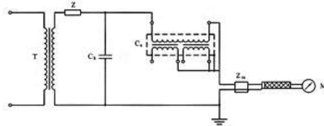
图 5.3 输入单元和电压互感器串接
