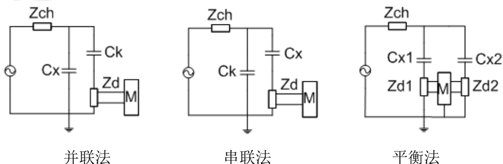
图 5.1 三种基本接法及优缺点
