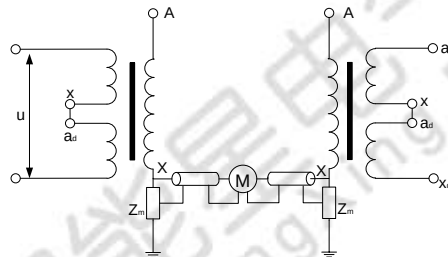
图 5.7 抑制干扰的平衡回路接线
