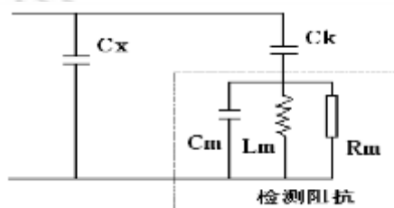
图 4.8 RLC 型输入单元的检测回路及等效电路示意图（并联法）
