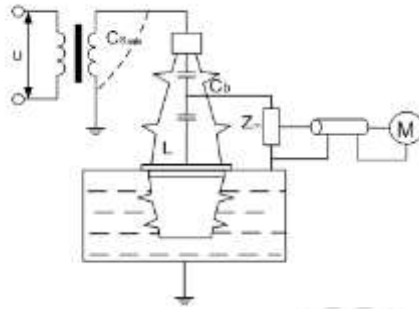
图 5.12 变压器套管接线
