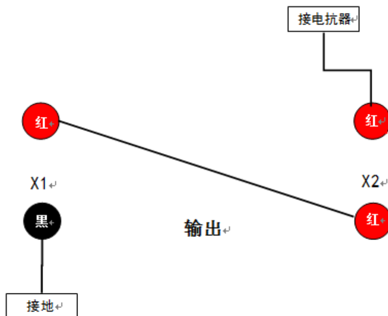
35KV 励磁变输出接线示意图
