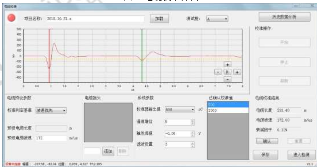
图 x 电缆校准界面
