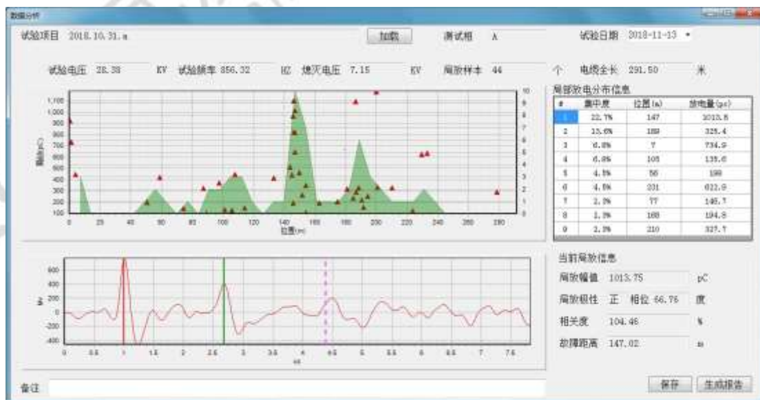
图 z 局放数据分析界面
