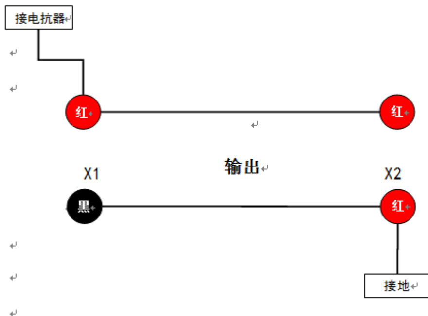
10KV 励磁变输出接线示意图
