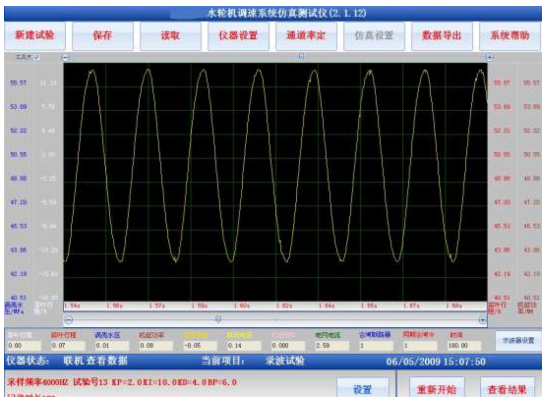
图 4.8 录波曲线
