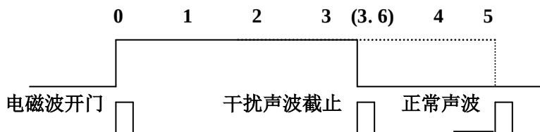
干扰声波误触发关系图
