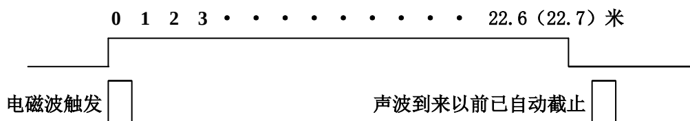
故障点较远或声波太弱时的关系图
