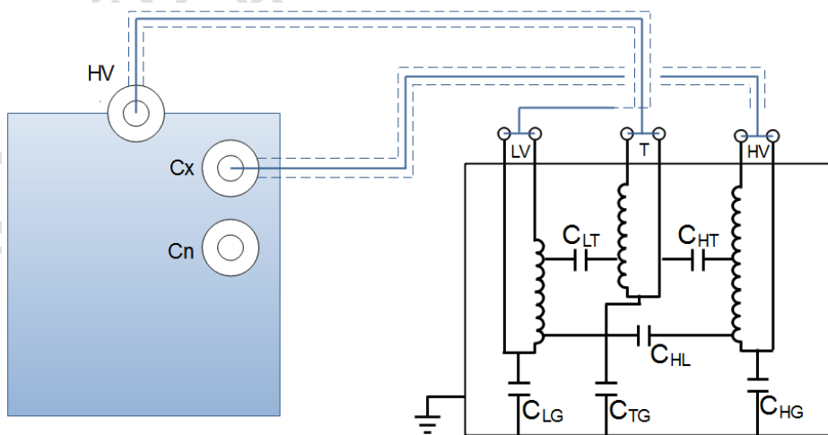
三绕组变压器 C_{TG}+C_{HT} (高压线屏蔽接 LV 绕组)
