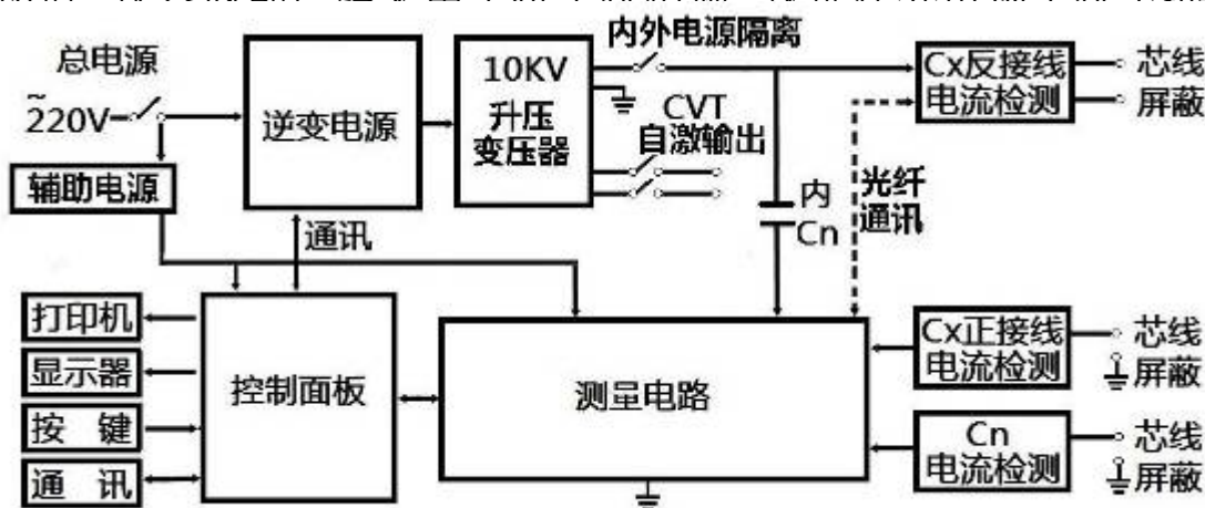
图 2—1 测量原理图
