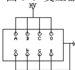
图 6-9 变压器接法
