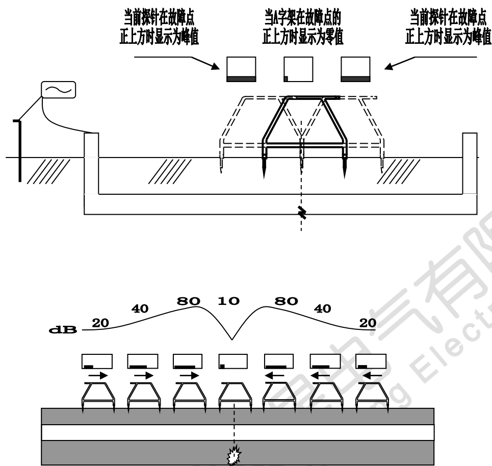
“A”字架探针在故障点处的信号显示
