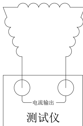
图十二 测量接线图
