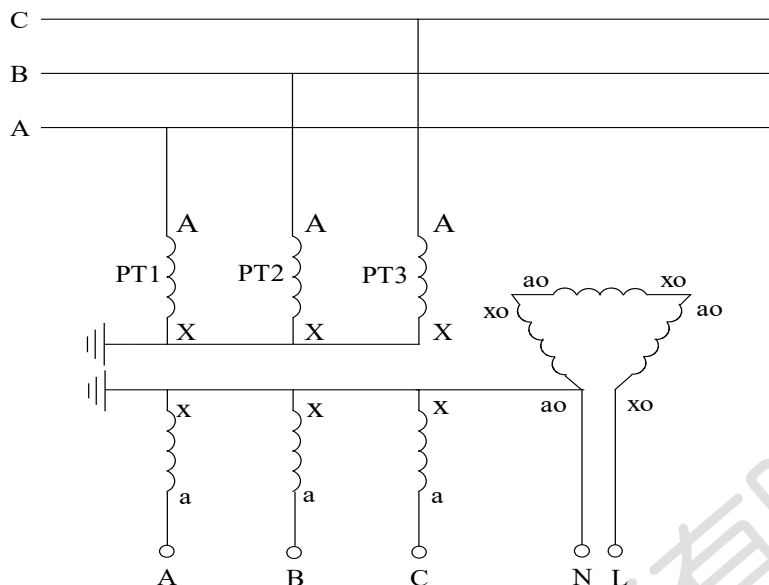
图四 N 接地方式
