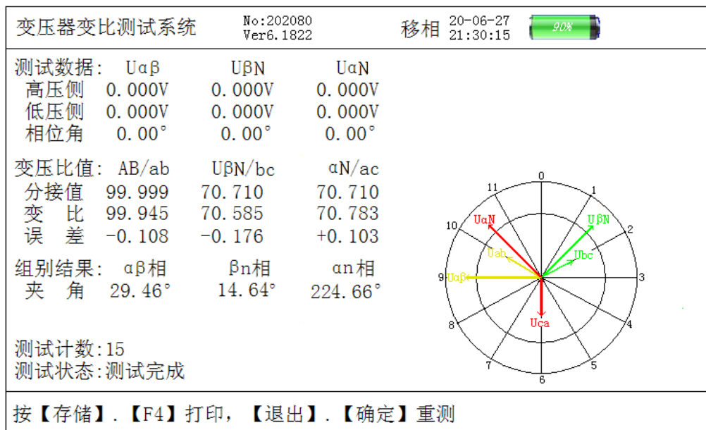
图十六、逆斯科特变压器测试结果屏
