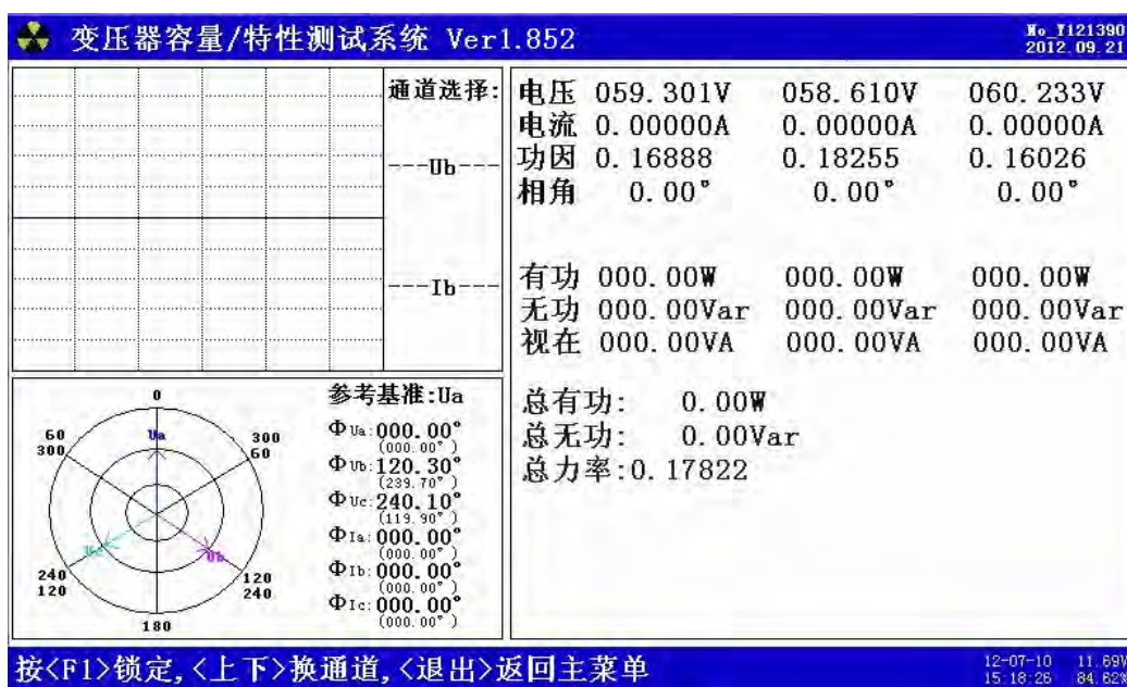
图 22、电气参量测量
