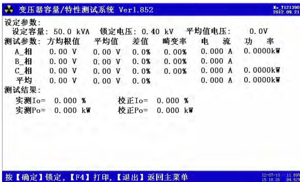
图 17、三相空载实时数据
