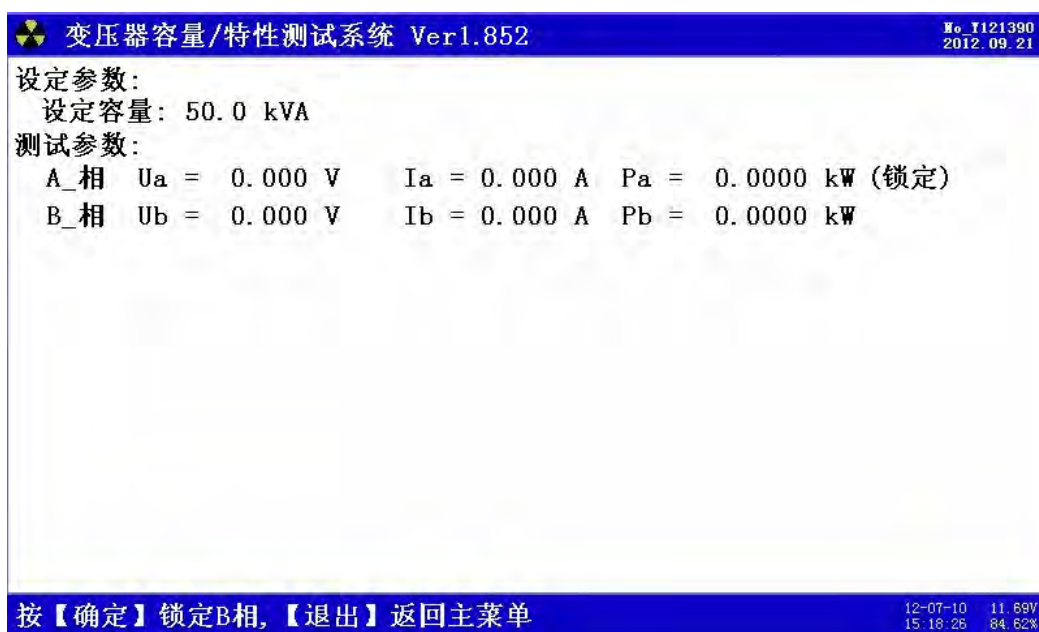
图 14、单相空载—B 相测量
