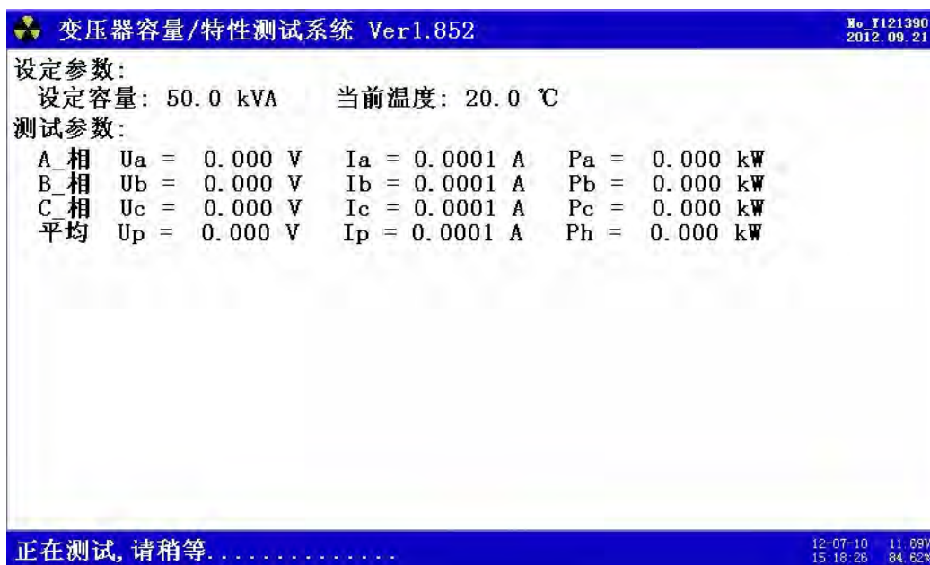
图 10、有源负载测试（进行中）
