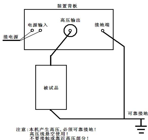
图 2 接线示意图（参考）
